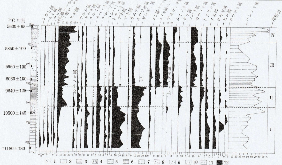
図30 鳥浜貝塚Ⅱ区(海拔0 m)の花粉ダイアグラム (出現率はハンノキ属をぬいた樹木花粉の総数を基数としてパーセントで表示)
